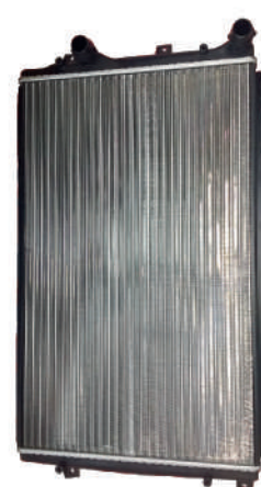
DRA0010301 VW GOLF V - AUDI A3 1.4i PANEL: 650X415X30 MM C/AC - S/AC
